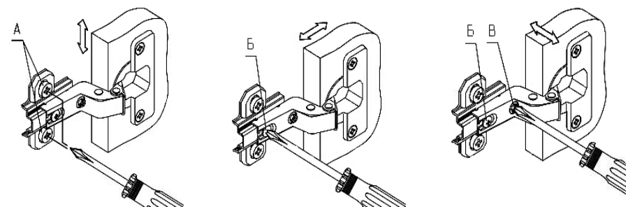
Схема 6. Регулирование положения фасада
