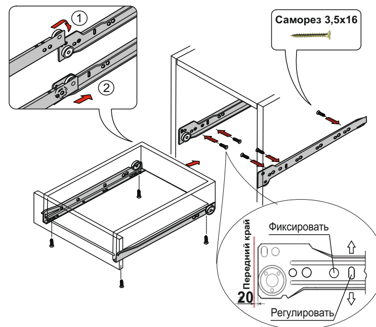
Схема 3. Установка направляющих
